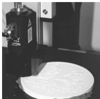
Bezdotykový přenos informace o reliéfu sádkového modelu.
