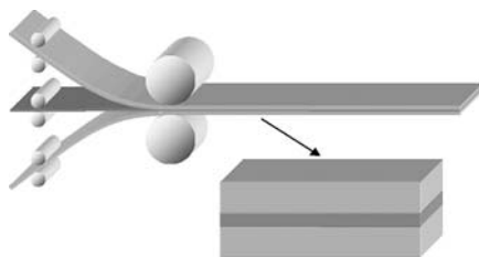
Zjednodušený princip plátování.
