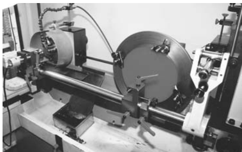
Moderní redukční stroj Bema 3001 v České mincovně.
