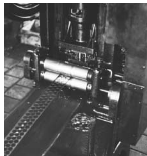
Střížky a zbývající cizura po průchodu cánů střížným zařízením.
